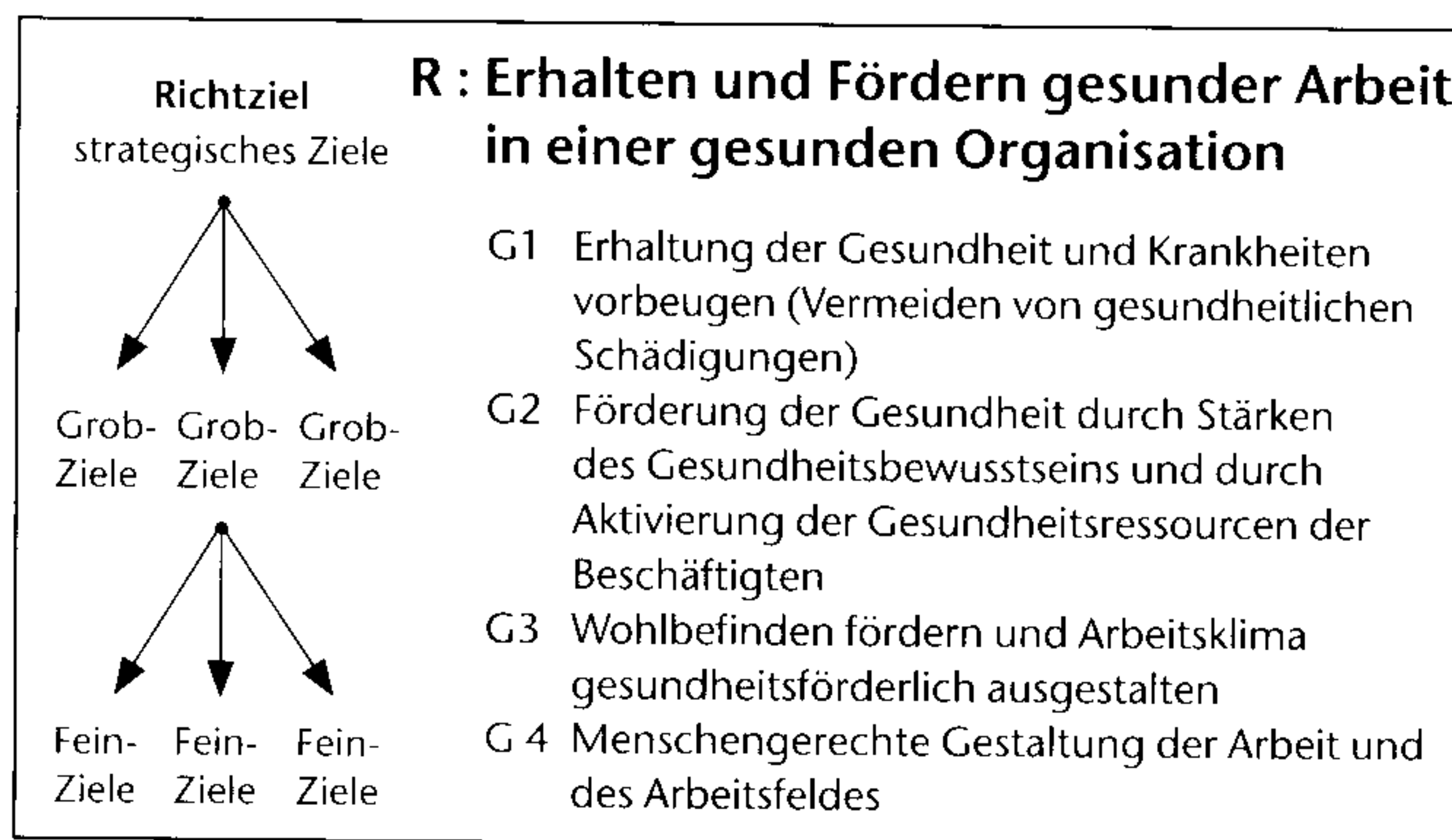
Abb. 5: Zielbaum Gesundheitsmanagement
